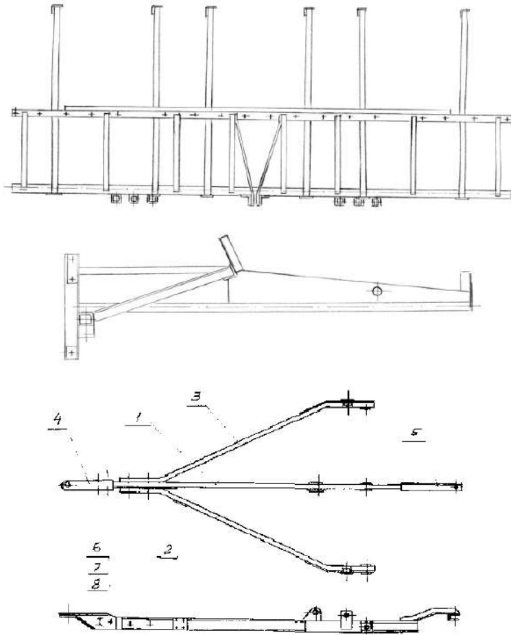
Рисунок 3 - Снпца в
