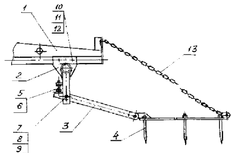
Рисунок 10 - Приспособление для навески борон (БЗСС-1,0 и цепь в базовую комплектацию не входят)
