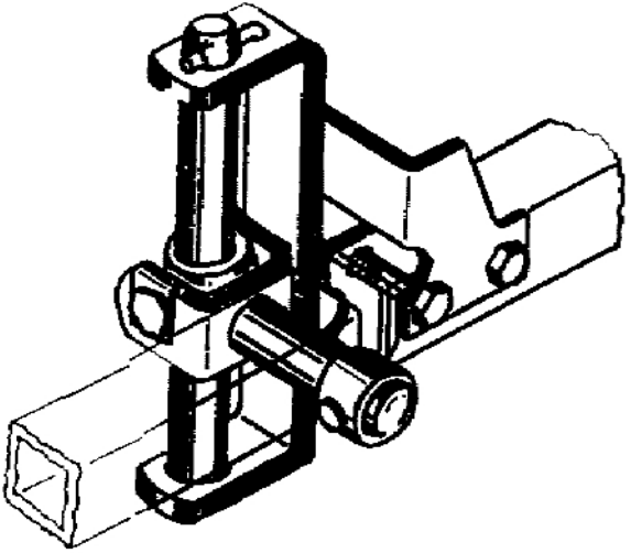
Рисунок 13 - Установка шарнира соединительного
