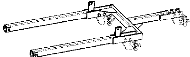
Рисунок 5-Грядиль обводной
