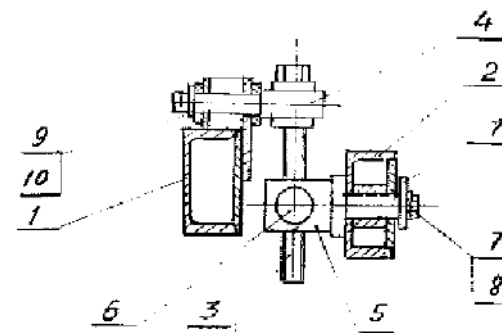
Рисунок 11 - Механизм регулировки глубины хода рабочих органов.
