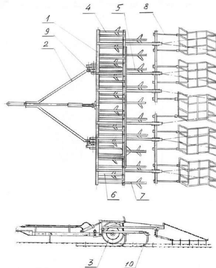
Рисунок 1 - Культиватор в сборе КСОП-5
